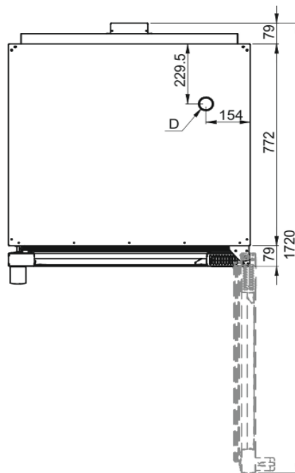
Vue du dessus porte ouverte
