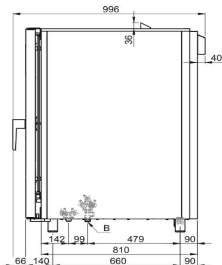
Vue côté
