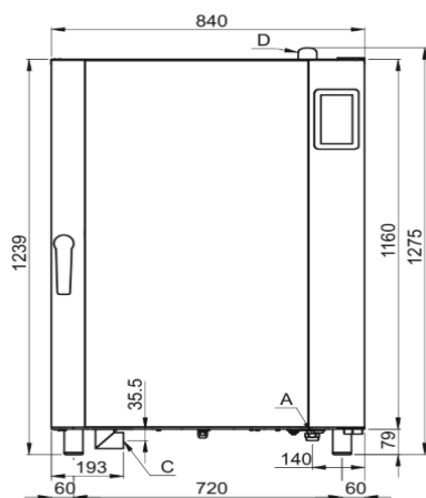
Vue face
